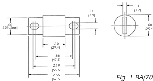
Fig. 1 BA(70A) – BL(250A)
