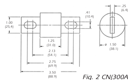
Fig. 2 CN(300A) – CZH(800A)
